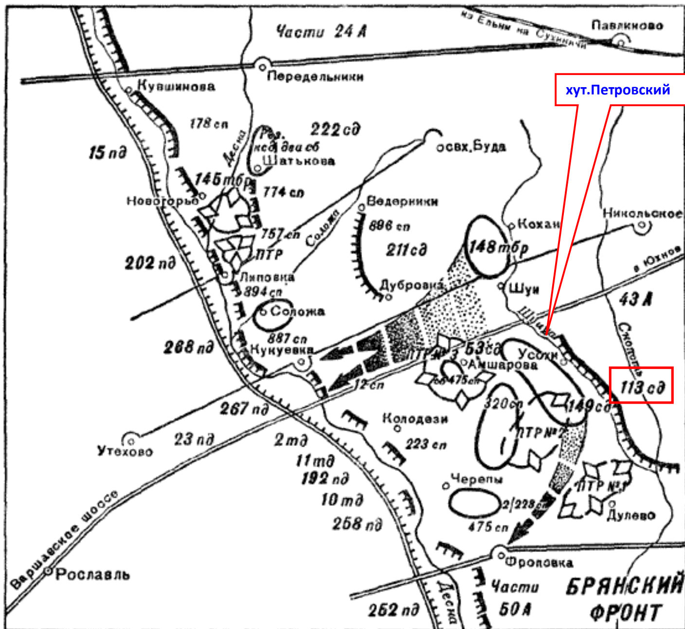
Построение обороны 43-й армии Резервного фронта на 1 октября 1941 г.
